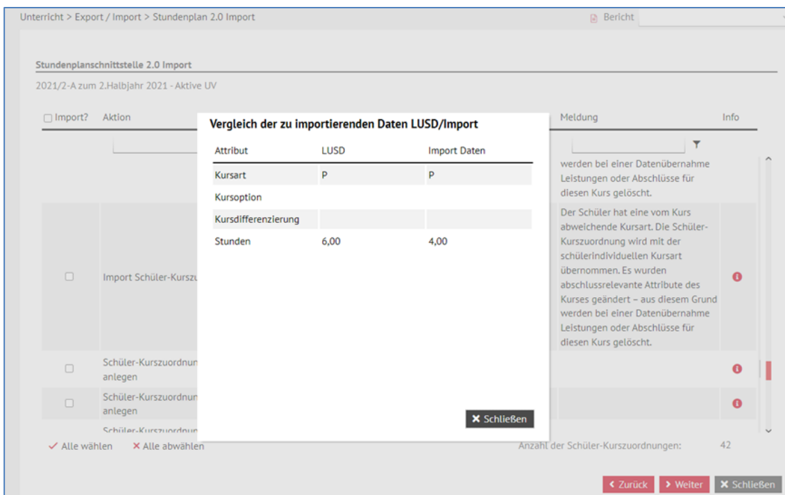
Abb. 8 Vergleich der zu importierenden Daten - Schüler-Kurszuordnung
