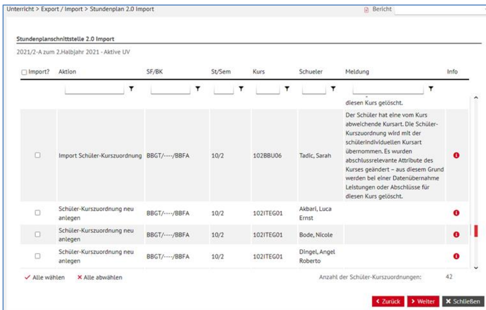
Abb. 7 Importassistent – Aktion Schüler-Kurszuordnung
